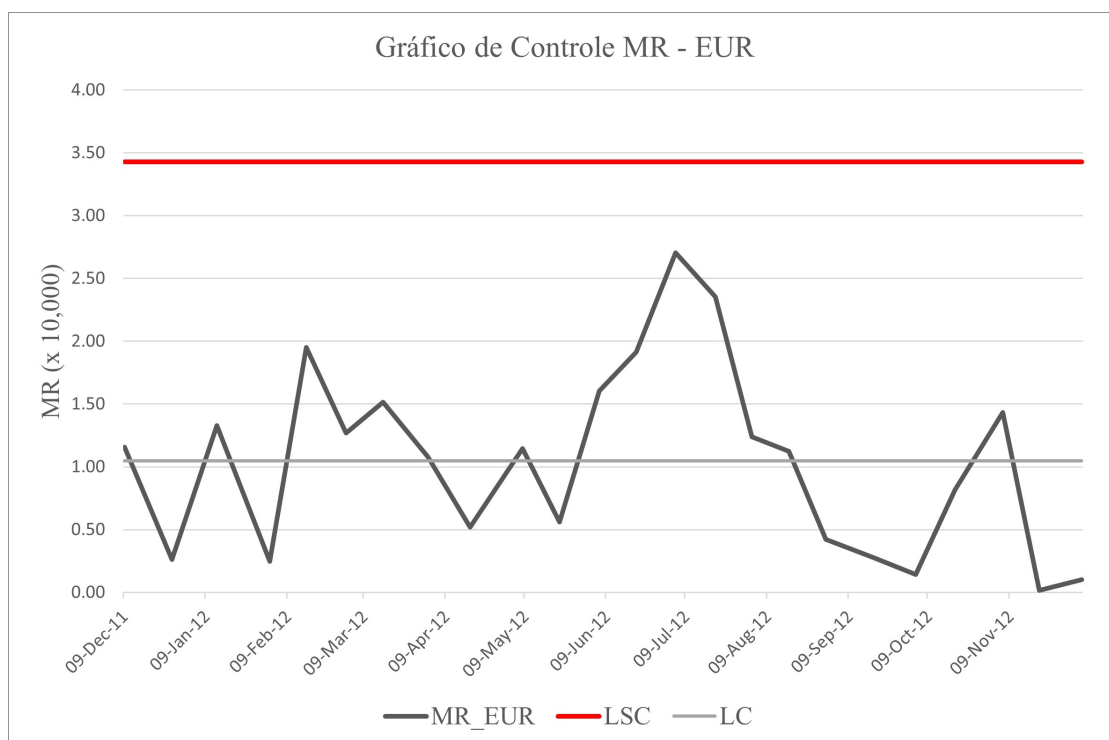
Figura 10 – Gráfico de Controle \overline{MR} para o Índice EUR
