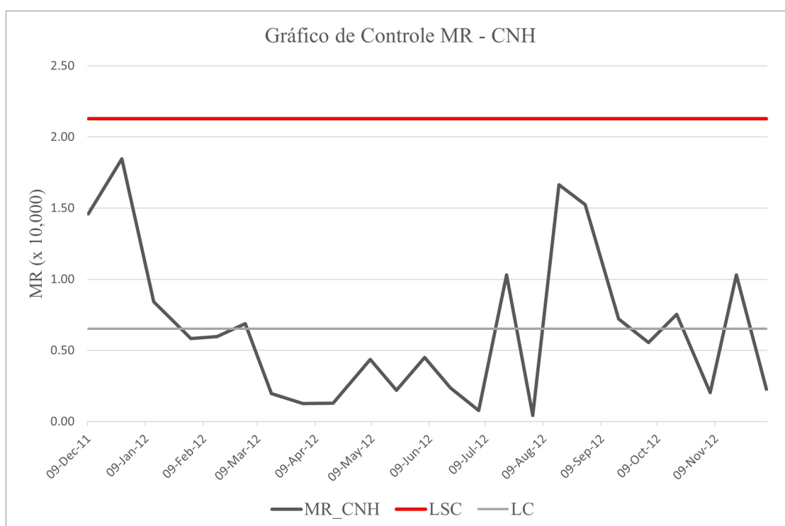
Figura 12 – Gráfico de Controle \overline{MR} para o Índice CNH
