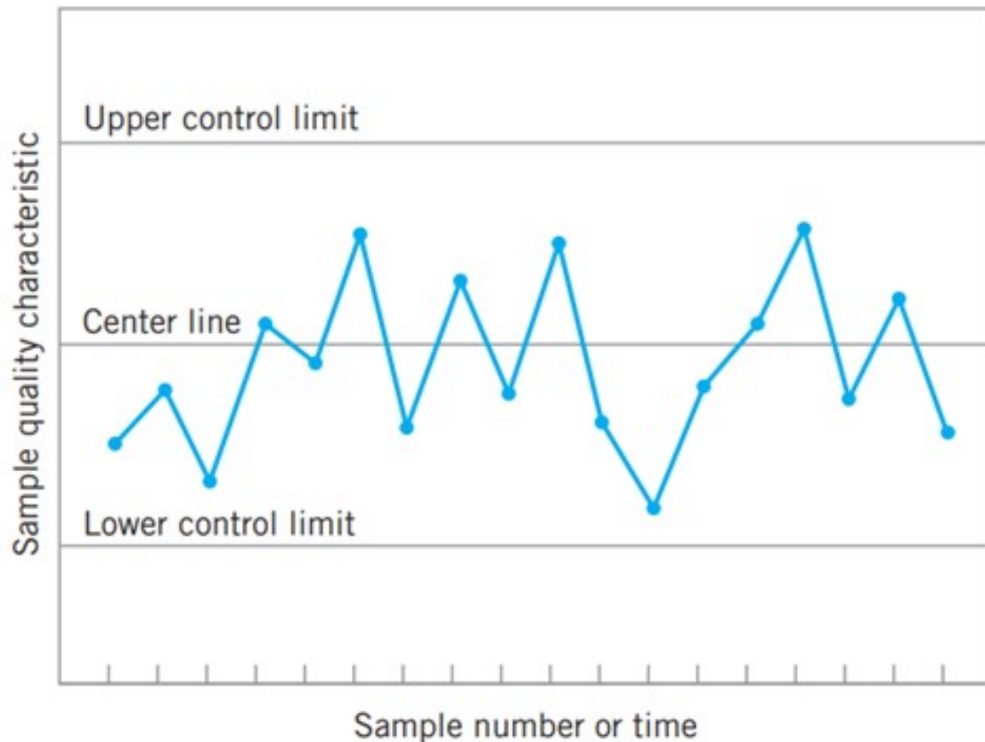
Figura 4 – Exemplo generalizado de um gráfico de controle
