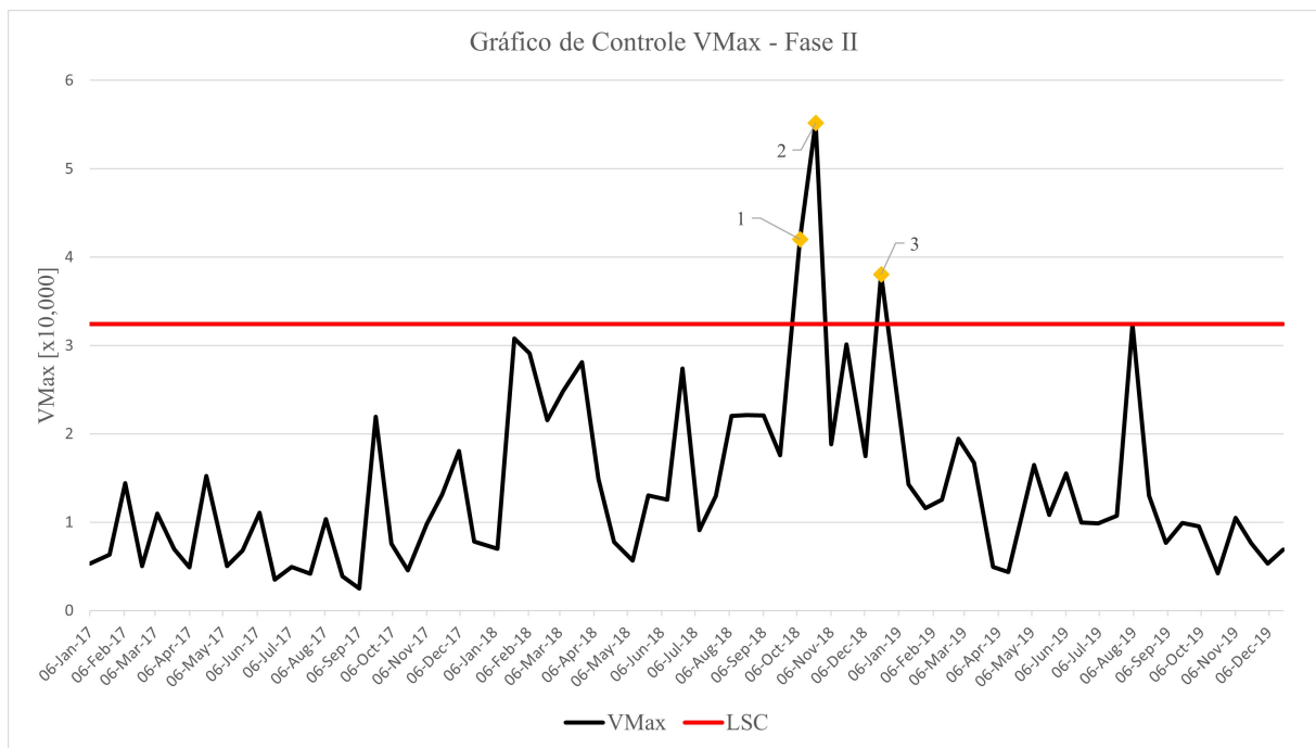
Figura 17 – Gráfico de Controle para VMax
