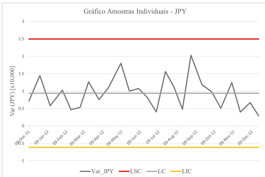
Figura 15 – Gráfico de Controle \bar{x} para o Índice JPY
