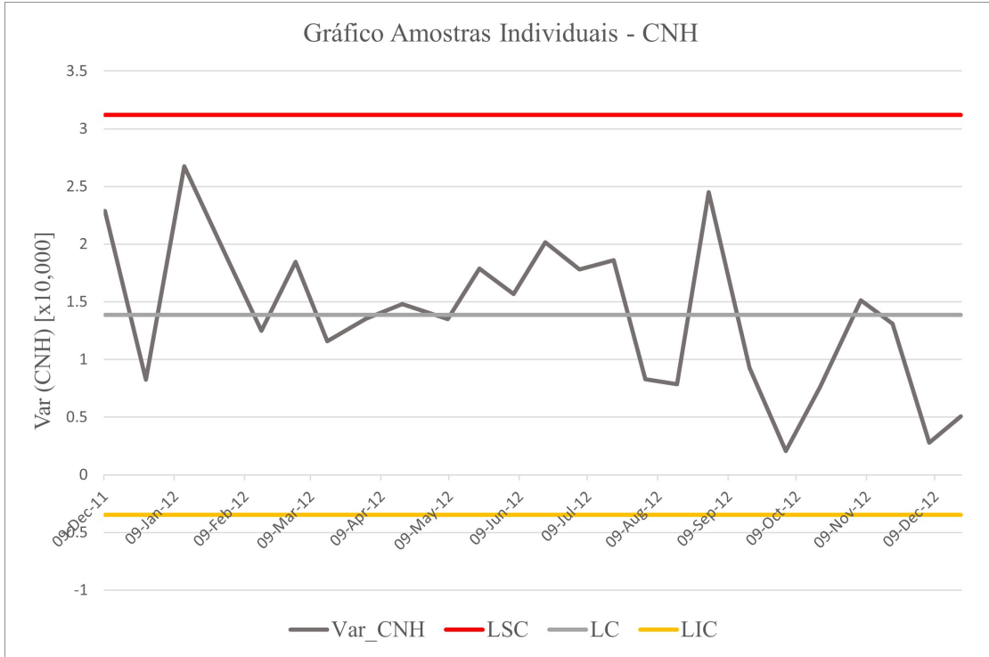
Figura 16 – Gráfico de Controle \bar{x} para o Índice CNH
