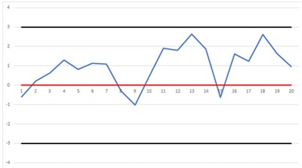
Figura 5 – Exemplo de comportamento fora de controle sem ultrapassar limites
