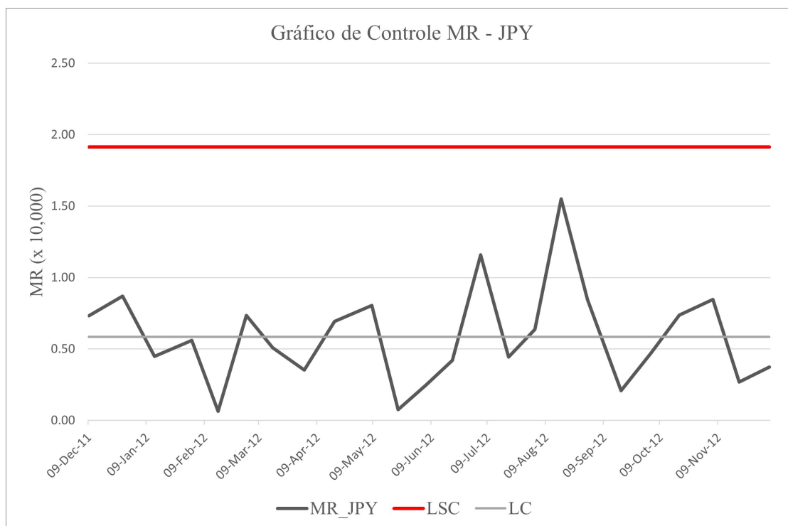
Figura 11 – Gráfico de Controle \overline{MR} para o Índice JPY
