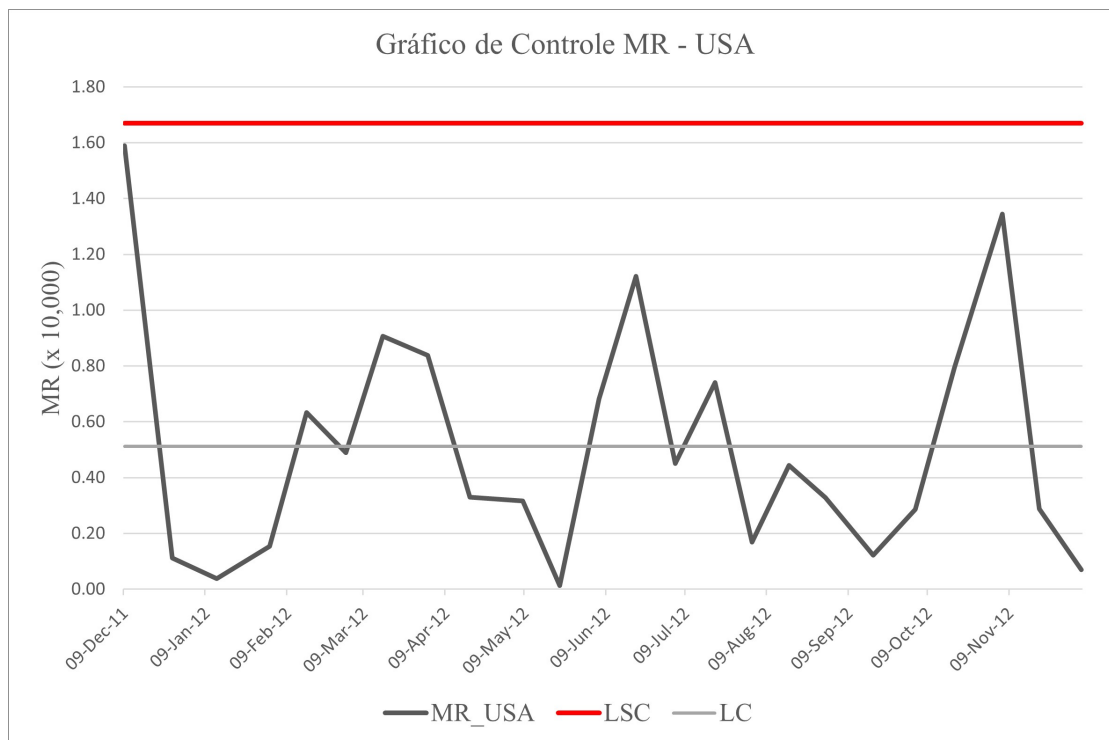
Figura 9 – Gráfico de Controle \overline{MR} para o Índice USA
