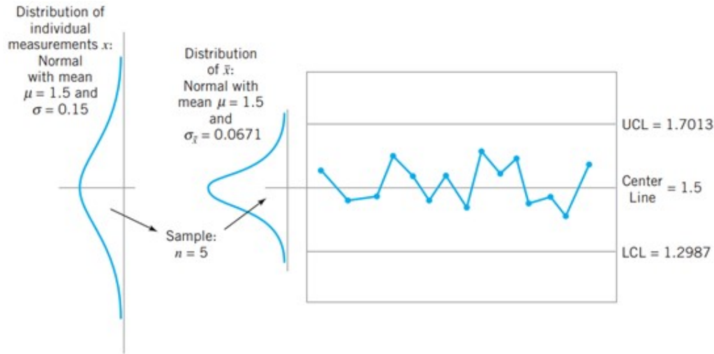
Figura 6 – Relação entre amostras, variável monitorada e gráfico de controle
